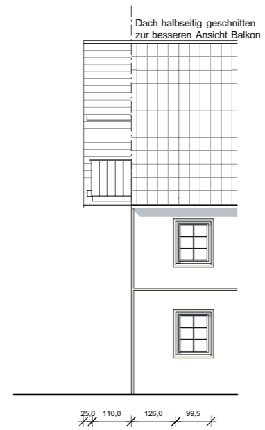
ANSICHT OST (Dach halbseitig geschnitten)
