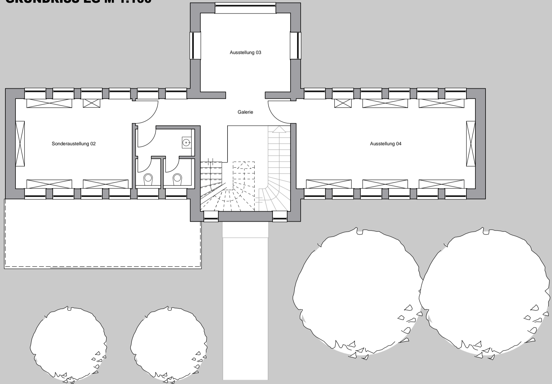
GRUNDRISS 1.OG M 1:100
