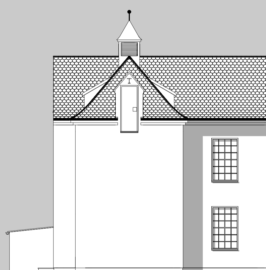
ANSICHT OST M 1:100
