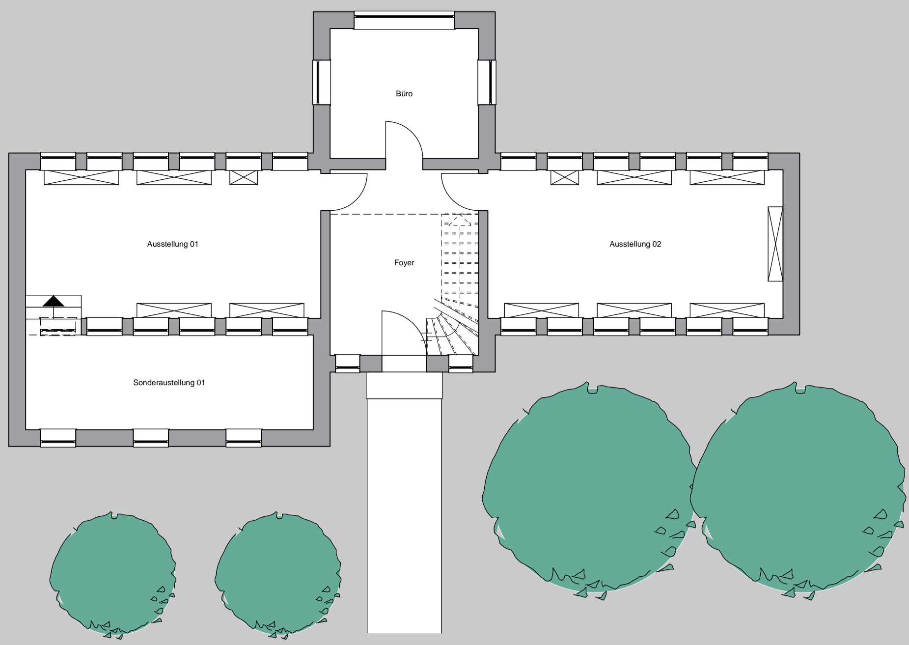
GRUNDRISS EG M 1:100
